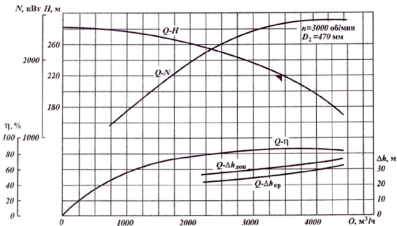
Рисунок А.10 – Рабочая характеристика насоса НМ 5000-210 со сменным ротором на подачу 3500 м³/ч
