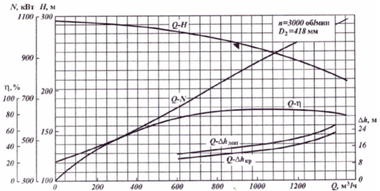
Рисунок А.1 – Паспортная характеристика насоса НМ 1250-260 со сменным ротором на подачу 900 м³/ч
