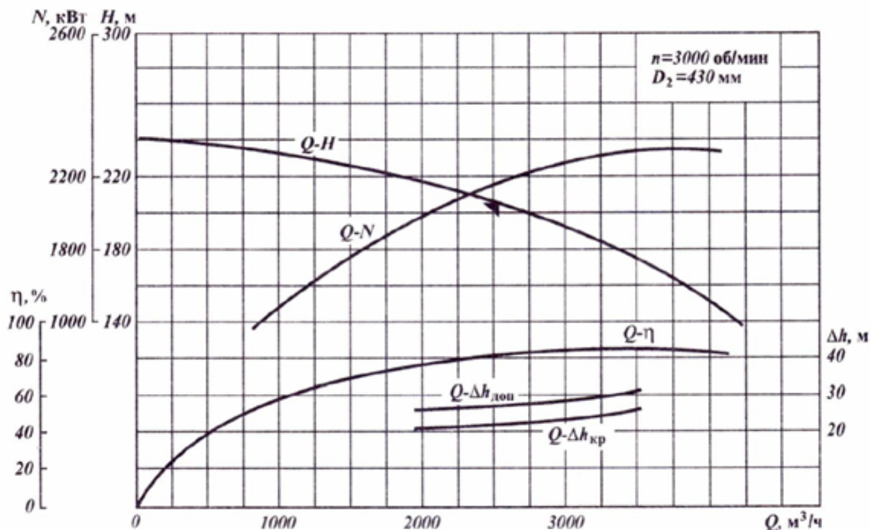
Рисунок А.9 – Рабочая характеристика насоса НМ 5000-210 со сменным ротором на подачу 2500 м³/ч
