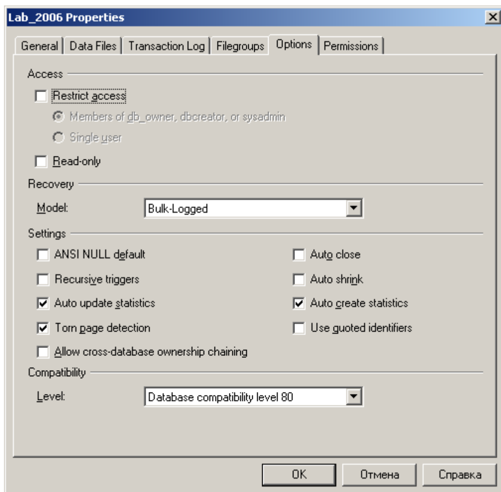
Рис 3.5. Вкладка OPTIONS
