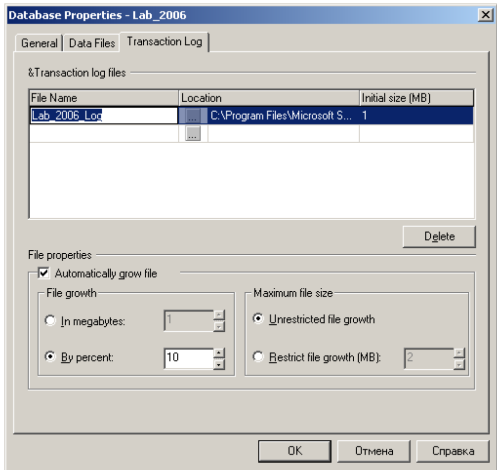
Рис 3.4. Вкладка Transaction_log
