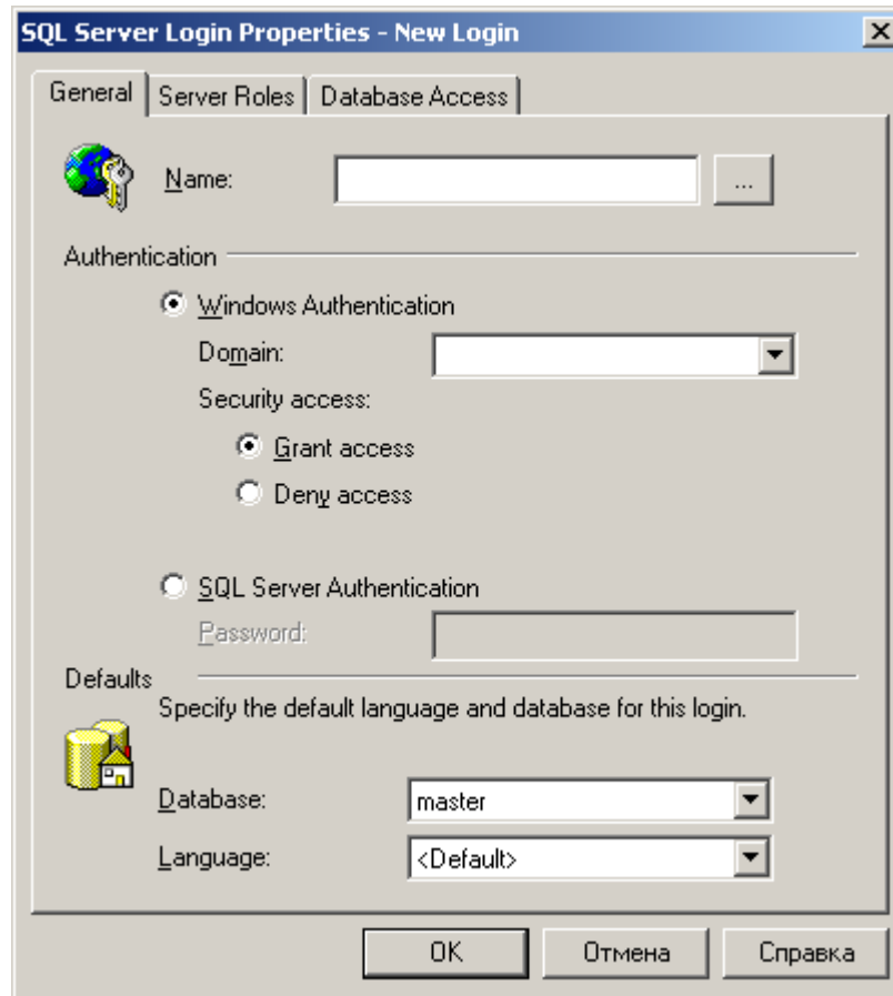
Рис 3.9. Вкладка General.
