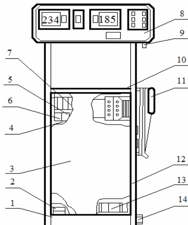
Рисунок 7 - Стойка приборная: 1 – шасси; 2 – блок зажимов; 3 – крышка; 4 – кассета; 5 – потенциометр P21; 6 – потенциометр P16; 7 – потенциометр P14; 8 – блок приборов; 9 – разъем выхода на ВУ; 10 – коврик; 11 – пульт дистанционного управления; 12 – силовой шкаф; 13 – разъем подключения опорного устройства; 14 – болт заземления.
