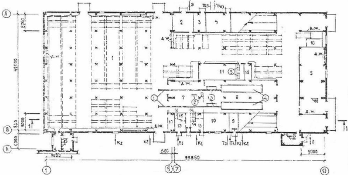
План на отм. 3.300
