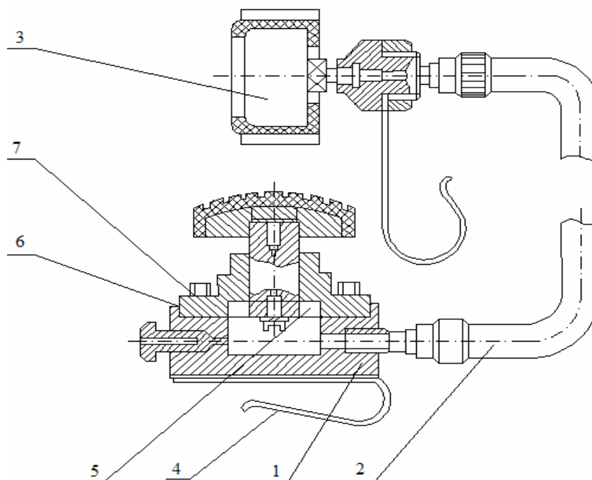
Рисунок 10 - Устройство силуизмерительное: 1 – корпус; 2 – трубка; 3 – манометр; 4 – захват пружинный; 5 – шток; 6 – крышка; 7 – мембрана
